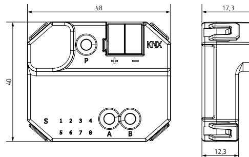
Coupleur de média TP-RF KNX
