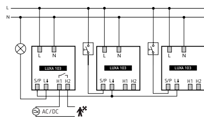
LUXA 103 S360-101, en montage en parallèle avec boutons-poussoirs
